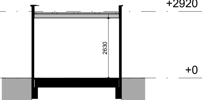
doorsnede A-A 1 : 100
