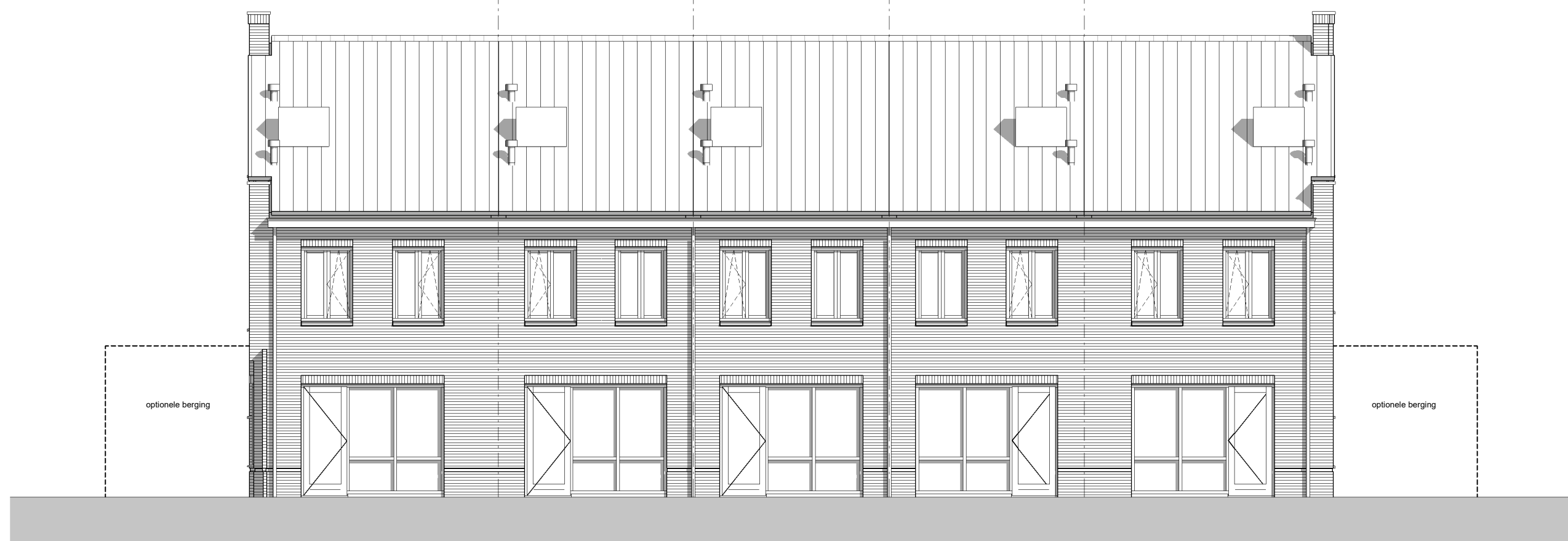
achtergevel 1:100
