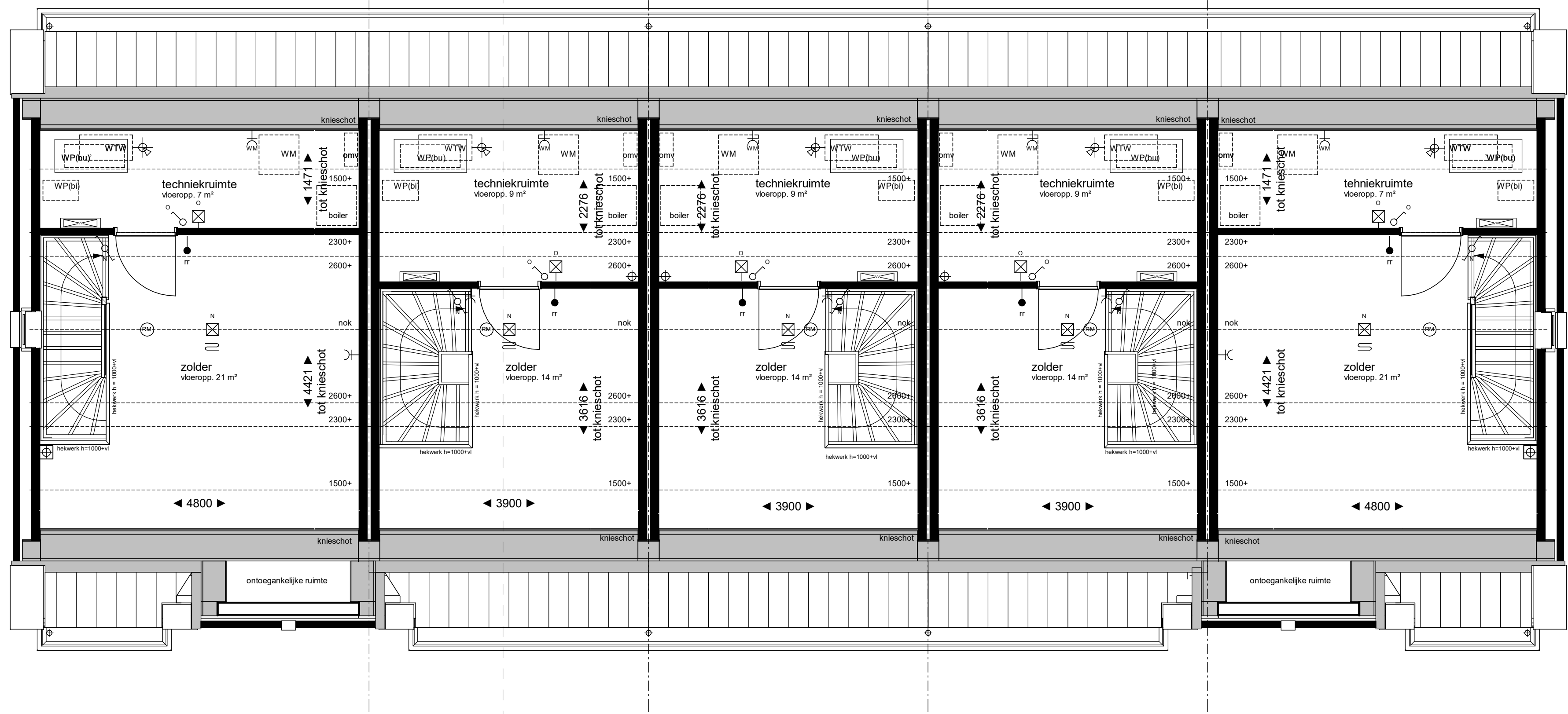
tweede verdieping 1:50
