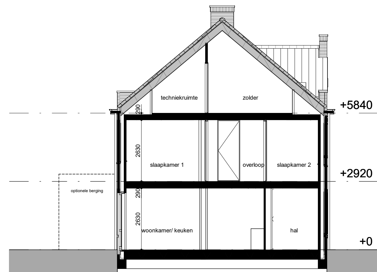
doorsnede AA 1:100
